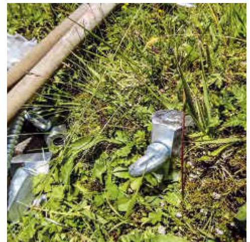
Anschlagpunkt im lockeren Schiefergestein. Eine 1,5 m lange Doka-Ankerstange wurde eingeschlagen. Den Abschluss bildet eine Spannmutter mit eingeschraubter Öse, eine Sonderanfertigung unseres Wasserwerks.
